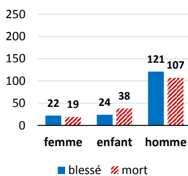
Statistiques des victimes au cours de Février 2017
