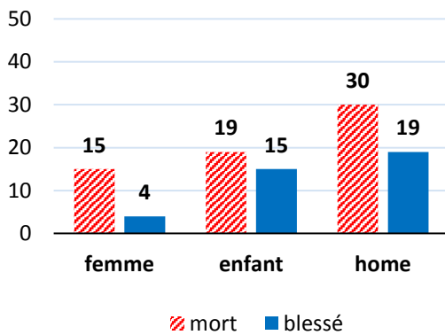
Statistiques de victimes au cours de mois de Février 2019
