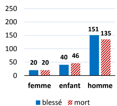
Statistiques des victimes au cours de Février 2018
