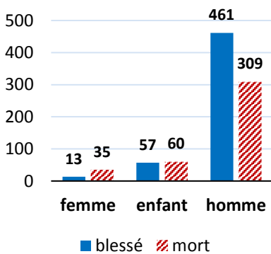
Statistiques des victimes au cours de Février 2016
